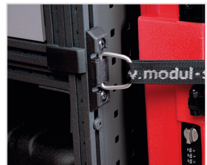
Befestigungsöse T-Nut
